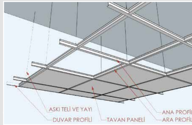
T24 Taşıyıcı Sistemi / T24 Load-Bearing System نظام الحمل ٤٢T
