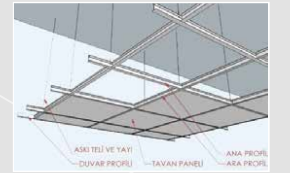
T24 Taşıyıcı Sistemi T24 Load-Bearing System نظام الحمل T24
